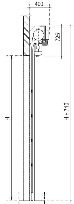
dwarsdoorsnede
