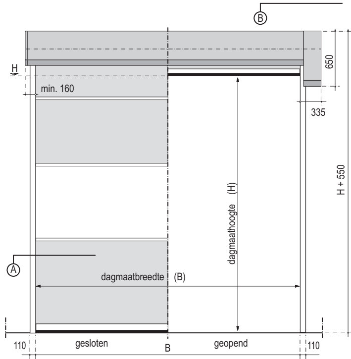
vooraanzicht
